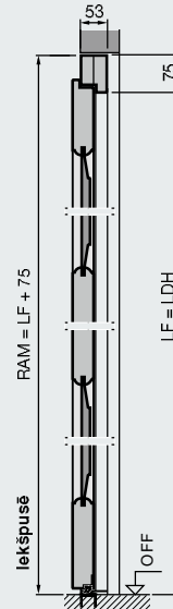
Sāna durvis no masīvkoka Montāža ailē
