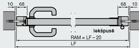
Sāna durvis ar alumīnija bloka kārbu, profila cilindrs 2 Montāža ailē
