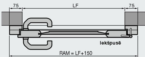
Sāna durvis no masīvkoka Montāža aiz ailes
