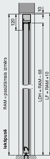
Sāna durvis ar alumīnija bloka kārbu, profila cilindrs 2 Montāža ailē
