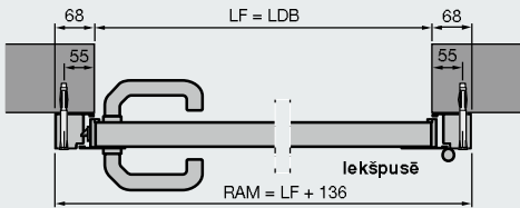
Sāna durvis ar alumīnija bloka kārbu, profila cilindrs 1 Montāža aiz ailes
