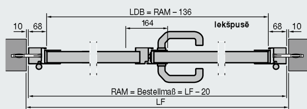
Divvērtņu sāna durvis ar alumīnija bloka kārbu, profila cilindrs 2 Montāža ailē
