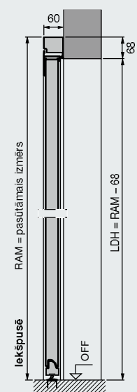
Sāna durvis ar alumīnija bloka kārbu, profila cilindrs 2 Montāža aiz ailes
