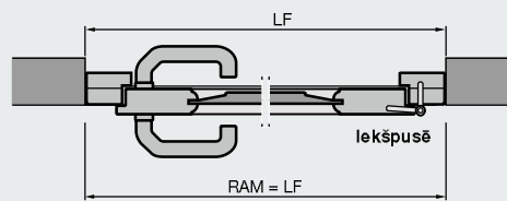
Sāna durvis no masīvkoka Montāža ailē
